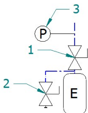
Obr 17 Zapojení expanzní nádoby
