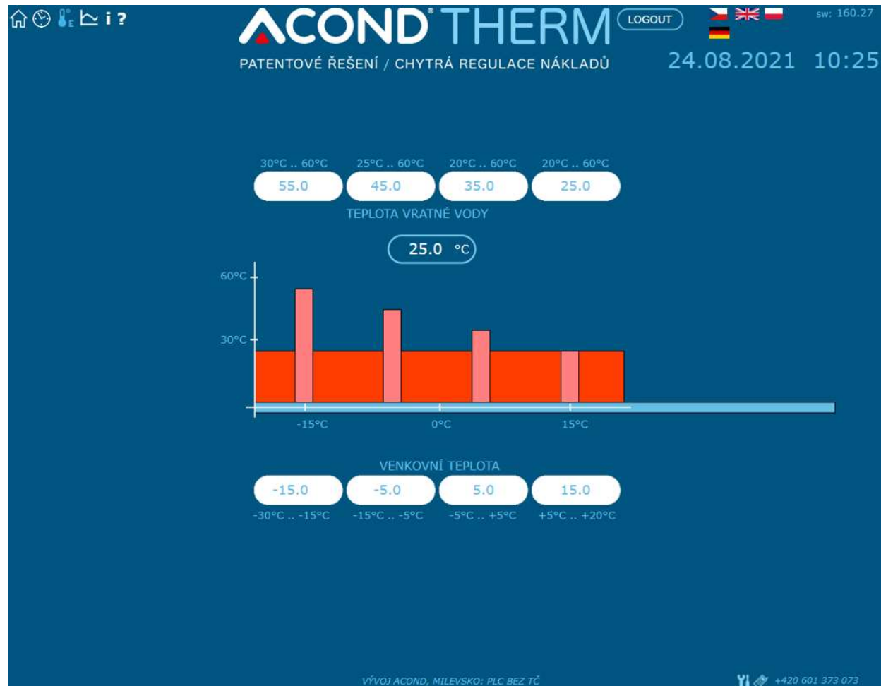
Obr 16 Nastavení ekvitermní regulace
